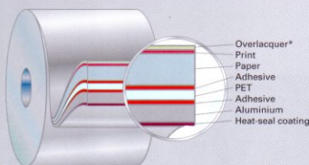
Peelable lidding
